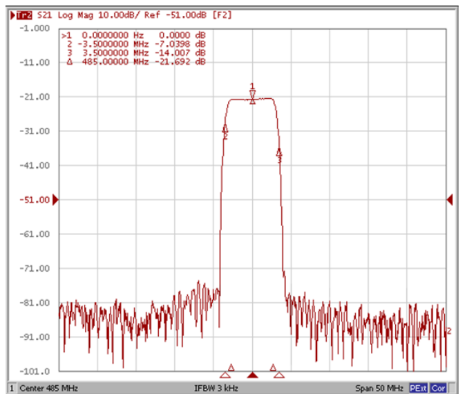
Attenuation (Fo±3.5MHz)
