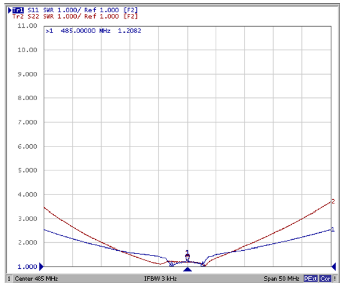
VSWR
